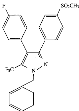
1-Benzyl-4-(4-fluorophenyl)-3-[4-(methylsulfonyl)phenyl]-5-(trifluoromethyl)pyrazole
