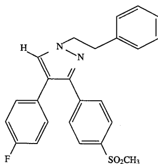
4-(4-Fluorophenyl)-3-[4-(methylsulfonyl)phenyl]-1-(2-phenylethyl)-1H-pyrazole
