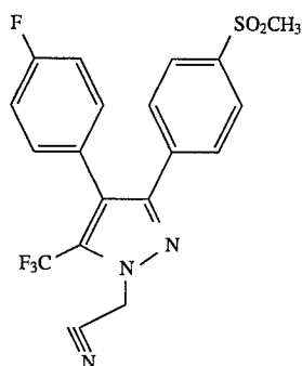
1-Cyanomethyl-4-(4-fluorophenyl)-3-[4-(methylsulfonyl)phenyl]-5-(trifluoromethyl)-1H-pyrazole
