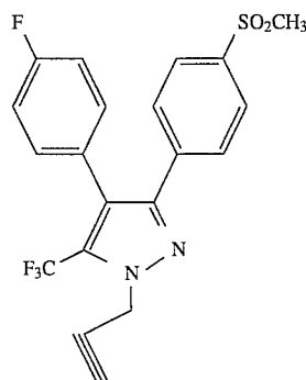
4-(4-Fluorophenyl)-3-[4-(methylsulfonyl)phenyl]-1-propargyl-5-(trifluoromethyl)-1H-pyrazole
