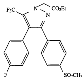
Ethyl[4-(4-fluorophenyl)-3-[4-(methylsulfonyl)phenyl]-5-(trifluoromethyl)-1H-pyrazol-1-yl]acetate
