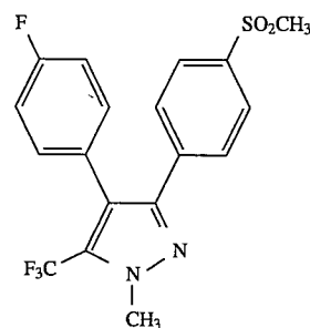
4-(4-Fluorophenyl)-1-methyl-3-[4-(methylsulfonyl)phenyl]-5-(trifluoromethyl)pyrazole
