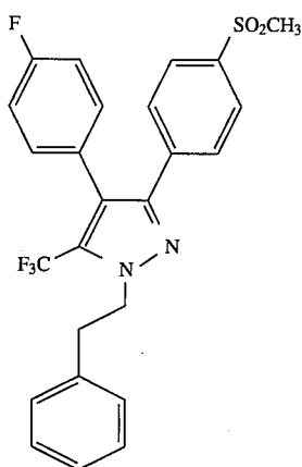
4-(4-Fluorophenyl)-3-[4-(methylsulfonyl)phenyl]-1-(2-phenylethyl)-5-(trifluoromethyl)pyrazole
