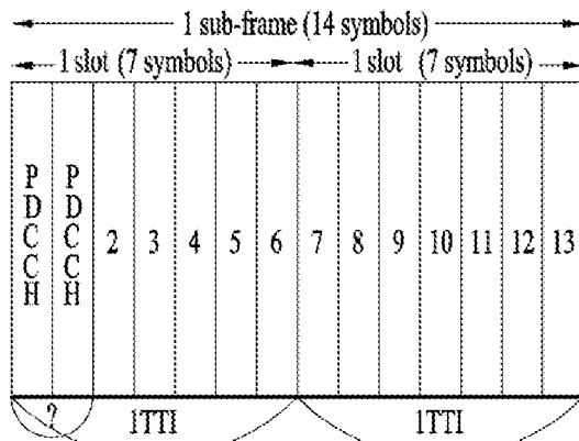
(d) 7 symbol TTI DL structure
