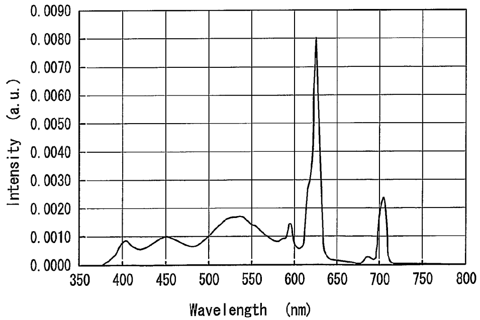
FIG. 52
