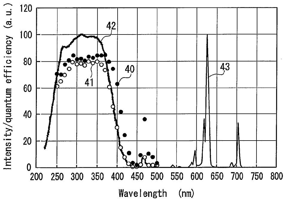
FIG. 40
