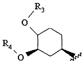
formule II
