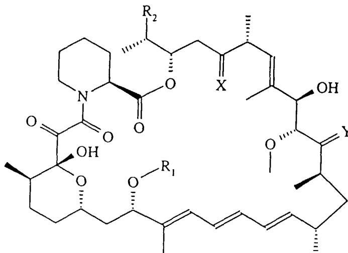
formule I
