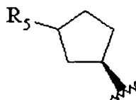
formule III
