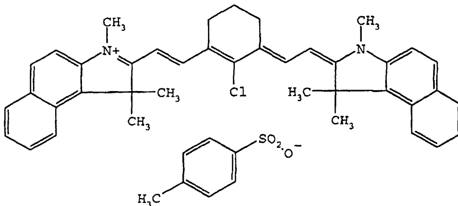
IR-absorber I
