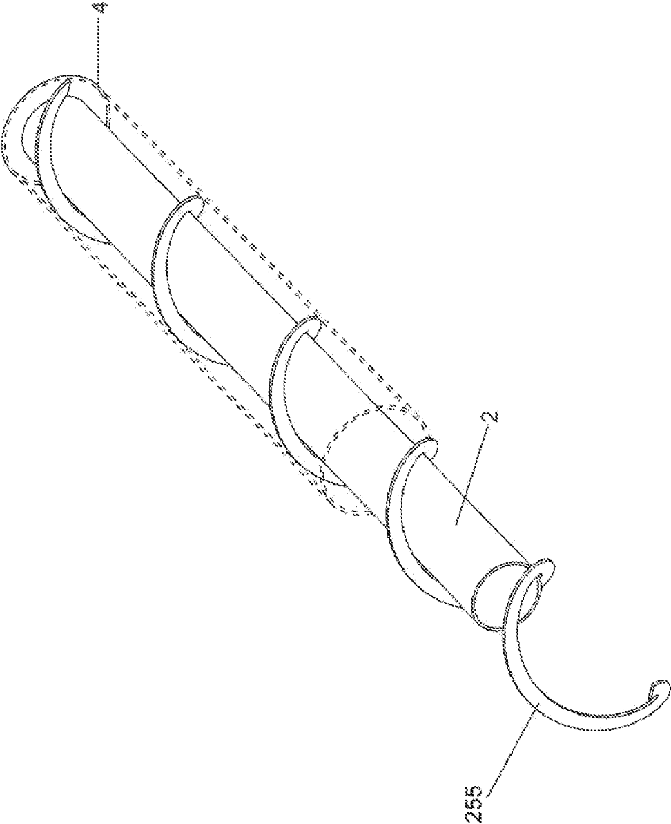
FIG. 115
