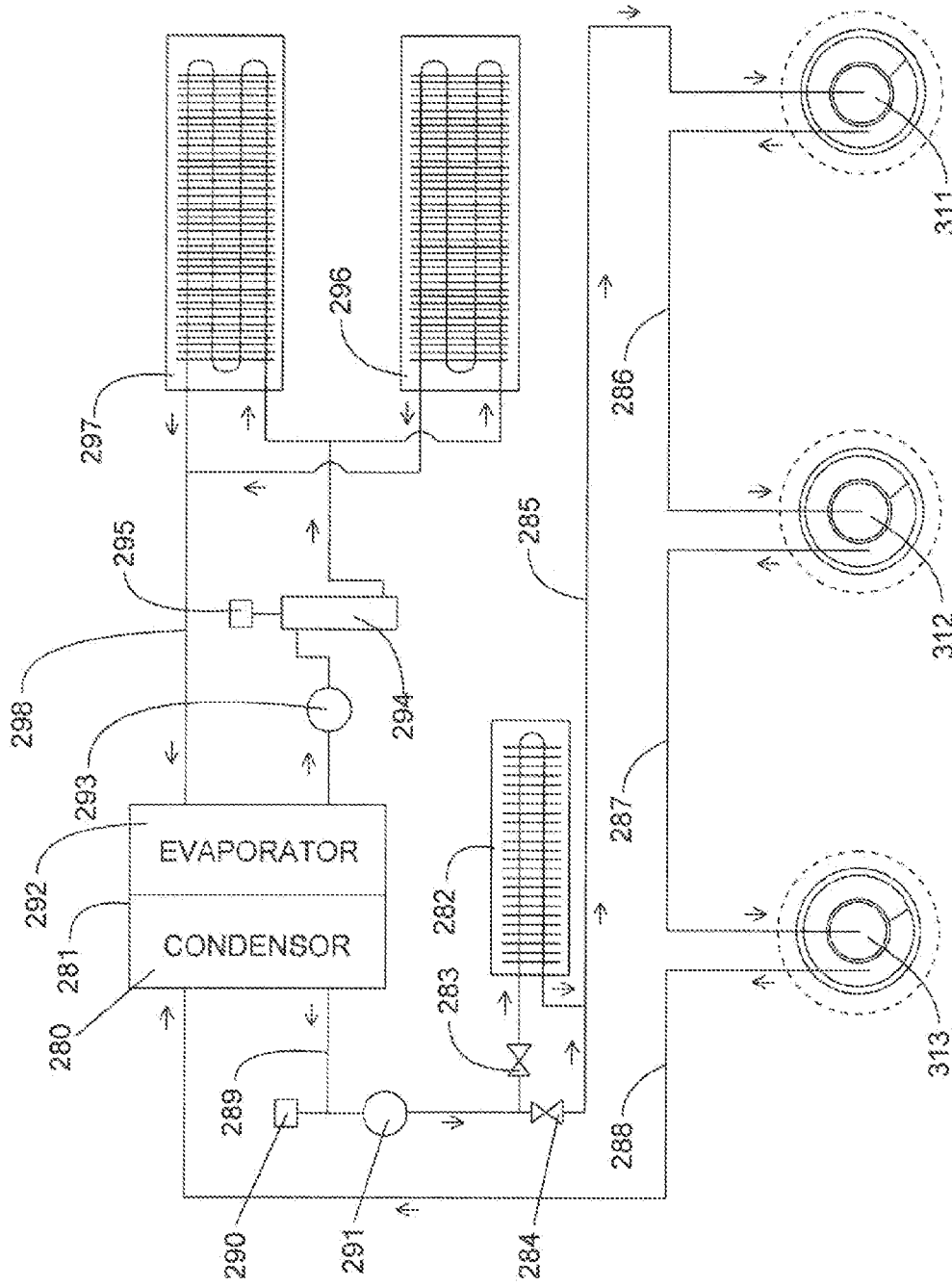
FIG. 119
