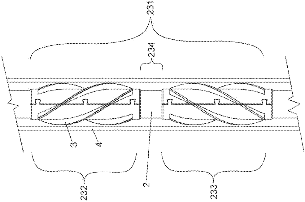
FIG. 103
